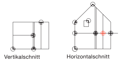
Vertikalschnitt
